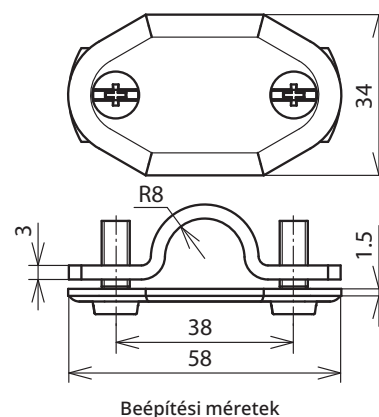
Beépítési méretek
