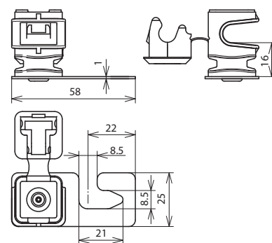
Beépítési méretek
