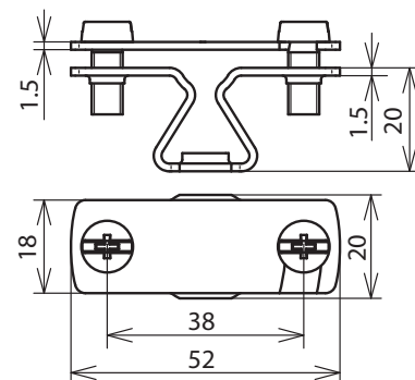
Beépítési méretek
