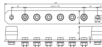
Beépítési méretek
