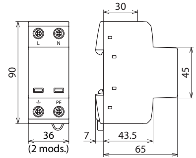
Beépítési méretek
