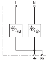
Kapcsolási rajz
