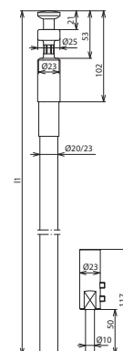
Beépítési méretek
