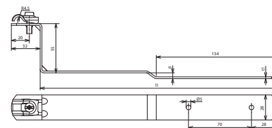
Beépítési méretek
