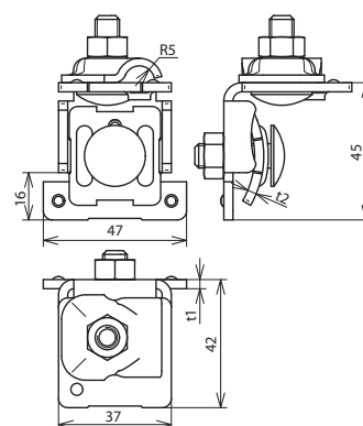
Beépítési méretek
