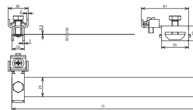
Beépítési méretek
