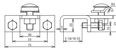
Beépítési méretek
