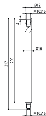
Beépítési méretek
