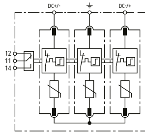
Kapcsolási rajz
