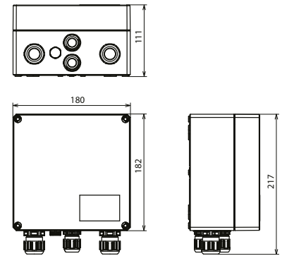
Beépítési méretek
