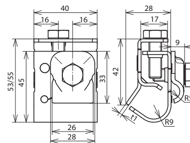
Beépítési méretek
