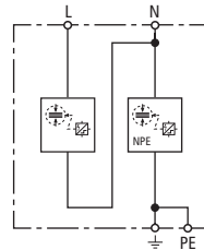
Kapcsolási rajz
