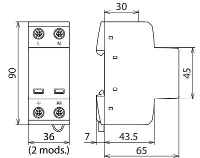
Beépítési méretek
