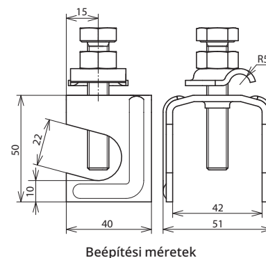
Beépítési méretek
