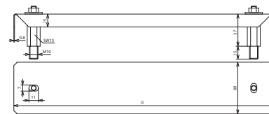
Beépítési méretek
