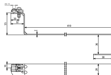
Beépítési méretek
