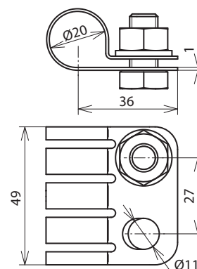
Beépítési méretek
