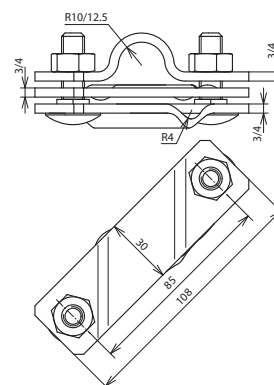
Beépítési méretek
