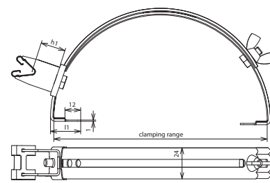
Beépítési méretek
