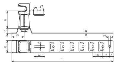
Beépítési méretek
