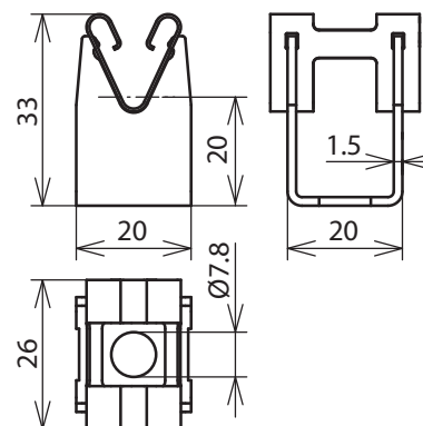
Beépítési méretek
