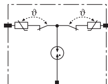
Kapcsolási rajz
