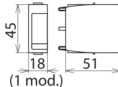
Beépítési méretek
