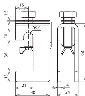
Beépítési méretek
