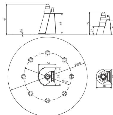
Beépítési méretek
