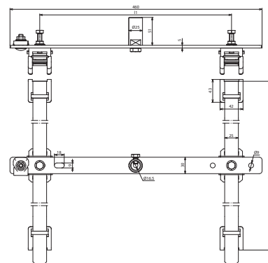
Beépítési méretek
