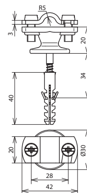
Beépítési méretek
