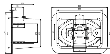
Beépítési méretek
