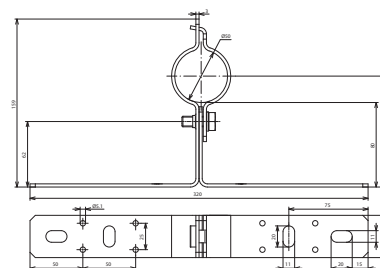
Beépítési méretek
