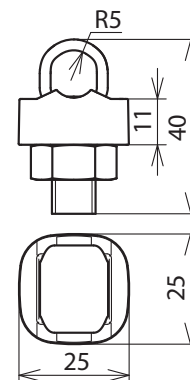
Beépítési méretek
