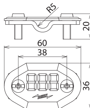
Beépítési méretek
