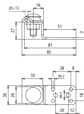
Beépítési méretek
