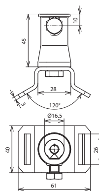
Beépítési méretek
