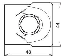
Beépítési méretek
