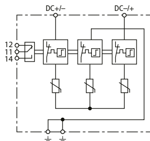
Kapcsolási rajz
