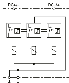
Kapcsolási rajz
