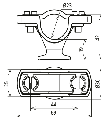
Beépítési méretek
