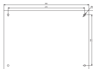
Beépítési méretek
