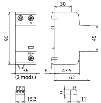
Beépítési méretek
