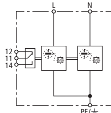
Kapcsolási rajz
