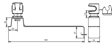
Beépítési méretek
