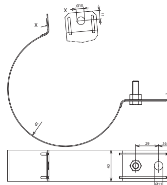
Beépítési méretek
