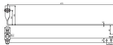
Beépítési méretek
