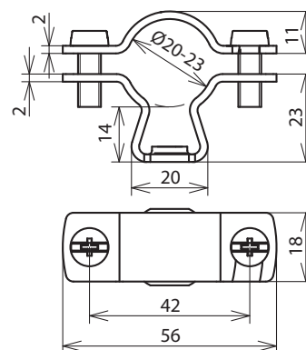
Beépítési méretek
