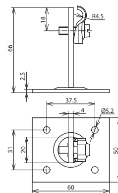
Beépítési méretek
