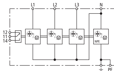
Kapcsolási rajz
