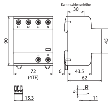
Beépítési méretek
