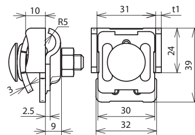
Beépítési méretek
