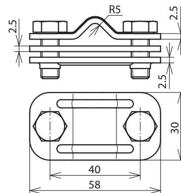
Beépítési méretek
