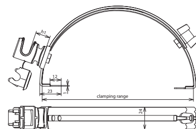
Beépítési méretek
