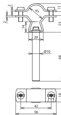
Beépítési méretek
