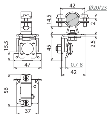
Beépítési méretek
